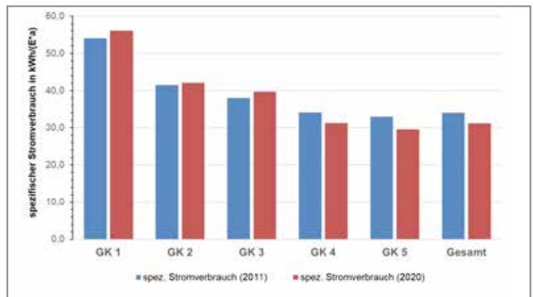
Abbildung 9: spezifische Stromverbräuche nach Größenklassen für die Jahre 2011 und 2020
